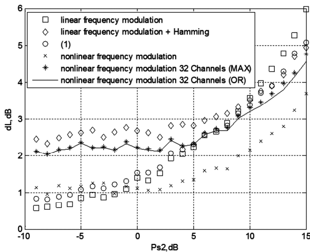
Рис. 4. Потери обнаружения
