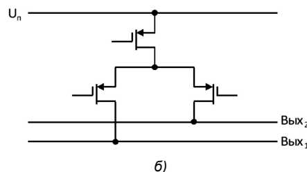
Рис. 1. Блок-схема N-разрядного ЦАП на источниках тока (а) и базовая ячейка такого ЦАП на КМОП-транзисторах (б): U n – напряжение питания; Вых1, Вых2 – токовые выходы
