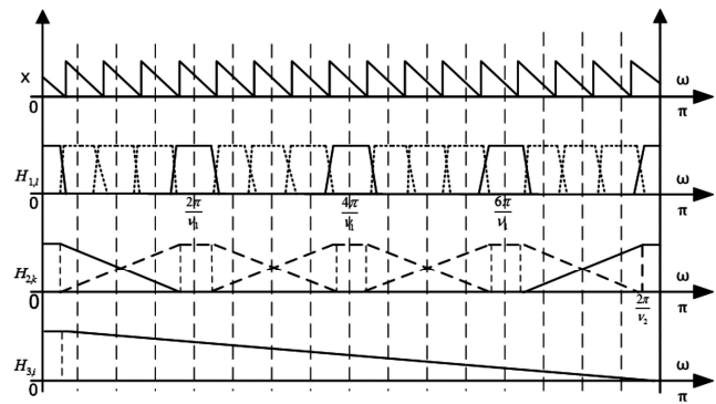
б) частотные характеристики каналов преобразования
