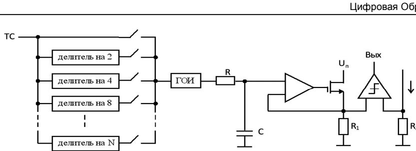
Рис. 2. Блок-схема, иллюстрирующая технику калибровки «весовых» токов: ТС – тактовый сигнал;
